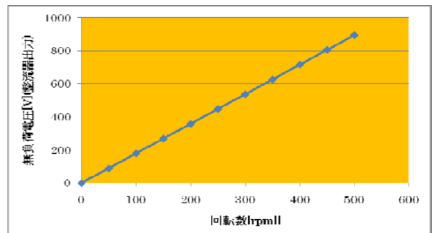
図 1 回転数－無負荷電圧特性
