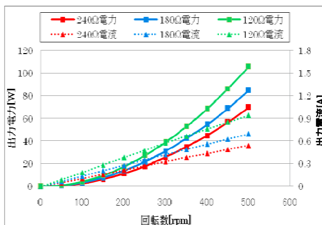
図 2 回転数 - 出力特性
