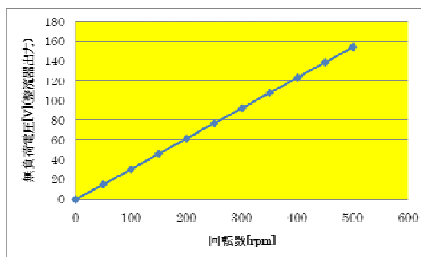
図 1 回転数 - 無負荷電圧特性
