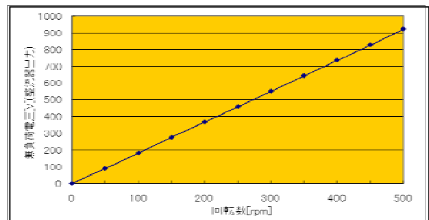
図1 回転数 - 無負荷電圧特性
