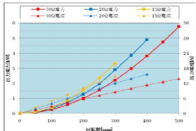
図2 回転数 - 出力特性
